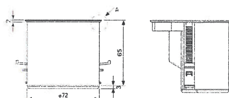
Découpe \phi 80 mm
