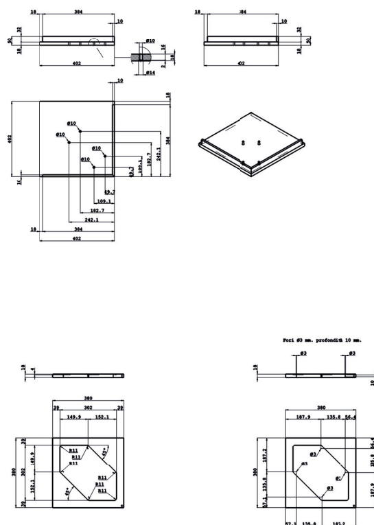
Particolare scasso da 4 mm.
